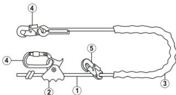
Рис. 7. Составные части стропа веревочного одинарного с регулятором длины ползункового типа «В11у»
